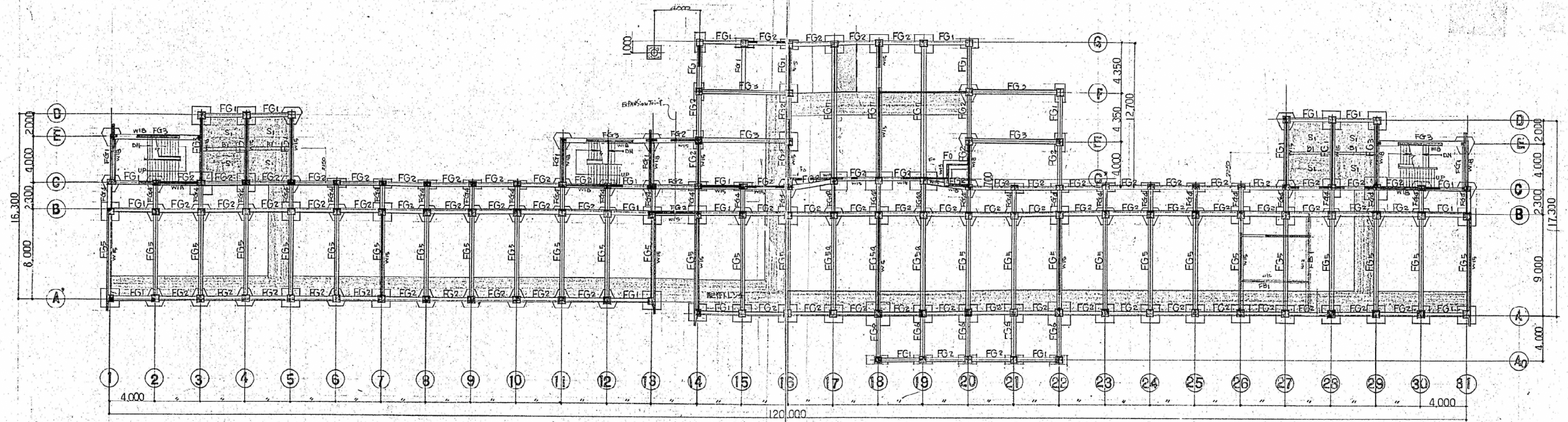
基礎伏図 1:200 特記事項参照 W12 とす
