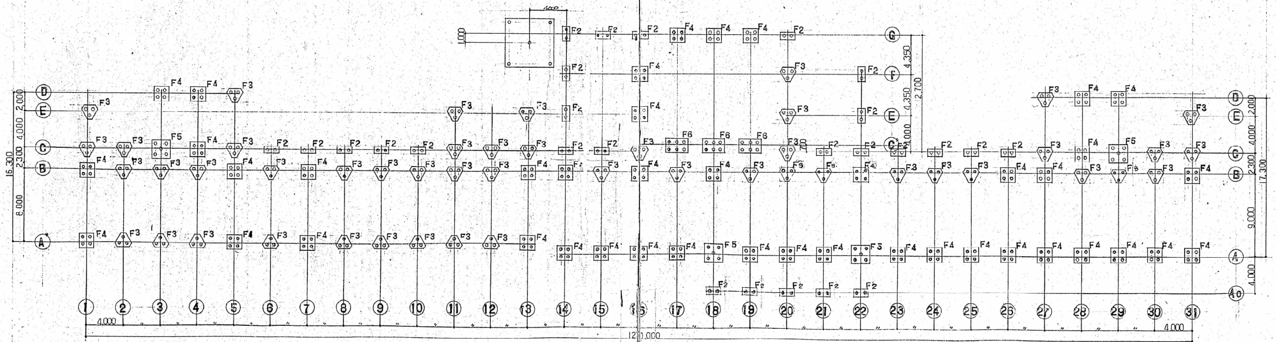
基礎伏図 1:200
