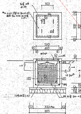
A排水樹断面図 1/20
