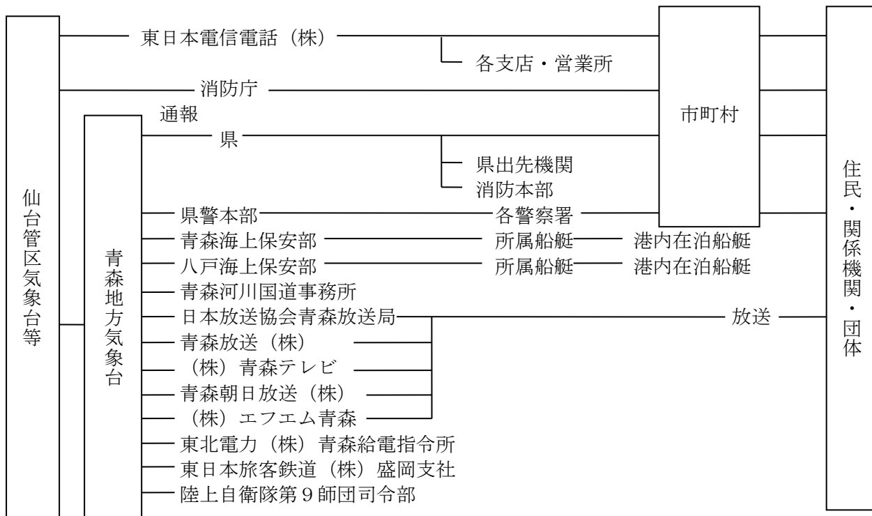
伝達系統図
