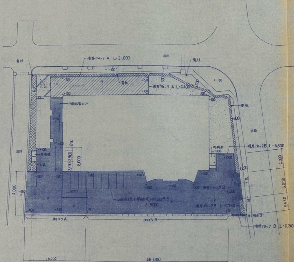
外構配置図 S:1/300
