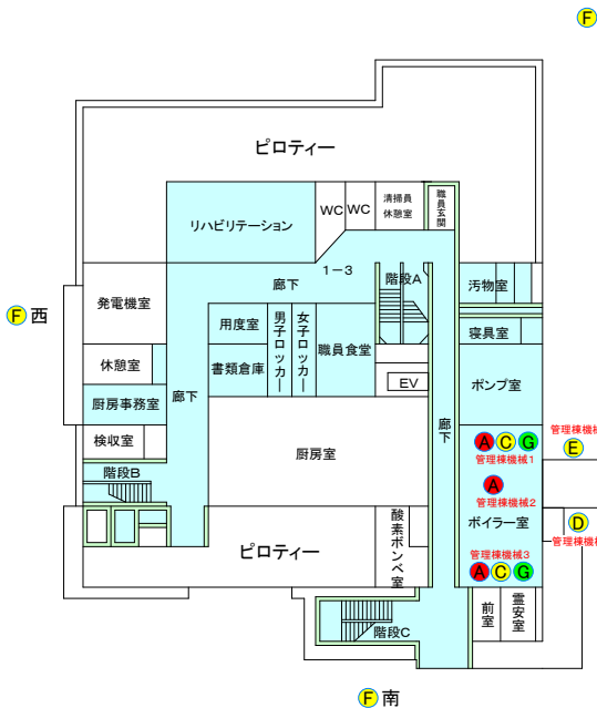
1階平面図
