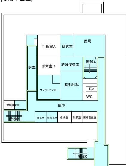
3階平面図
