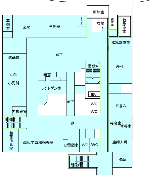
2階平面図
