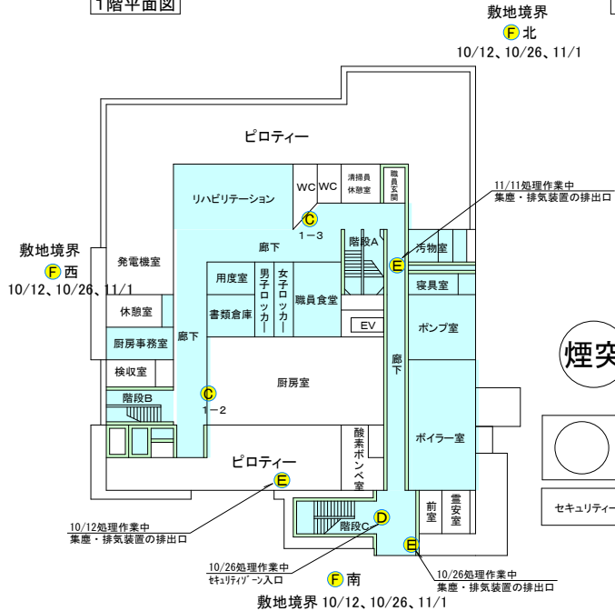
1階平面図
