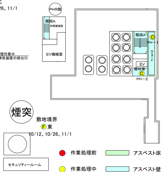
PH階平面図
