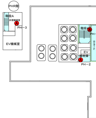
PH階平面図
